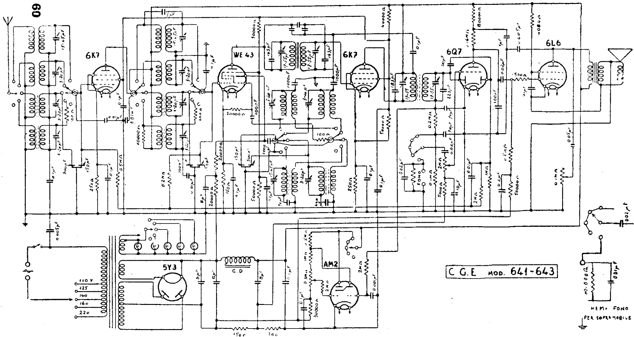
COMPAGNIA GENERALE DI ELETTRICITÀ. — Mod. 641 e 643 radiofonografo. — Produzione 1938-39. — Media frequenza: 459 kHz.
